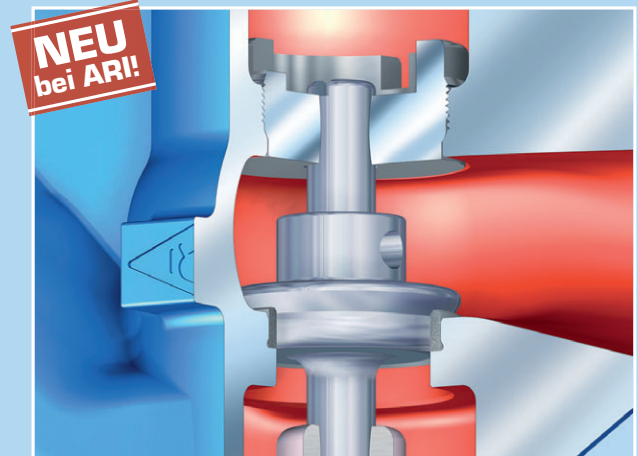
Thermo-Öffnungsventil (für Kühl-Systeme) öffnet mit steigender Temperatur
