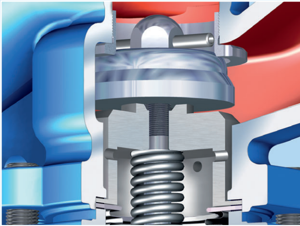
Thermo-Schließventil (für Heiz-Systeme) schließt mit steigender Temperatur
