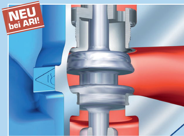
Thermo-Mischventil (für Misch- und Verteil-Systeme) reduziert bzw. schließt Eingang B bei steigender Temperatur
